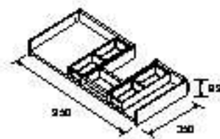
CAJÓN METÁLICO CON SALVASIFÓN IZQUIERDO
