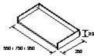
CAJÓN METÁLICO COMPLETO SIN SALVASIFÓN
